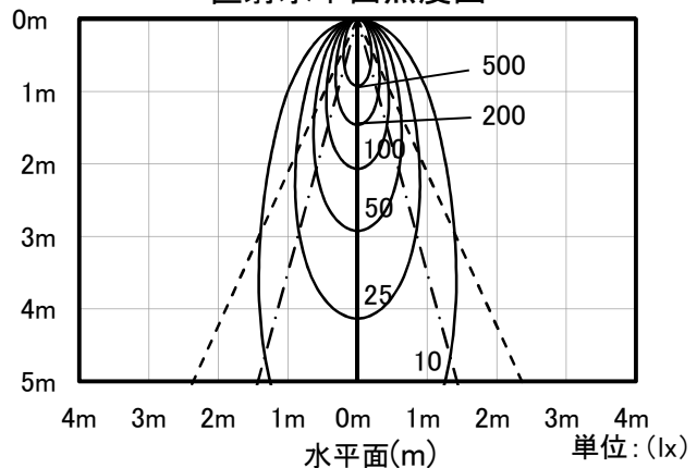
直射水平面照度図 初期値
