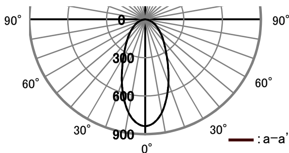
配光曲線 (cd/1000[lm])
