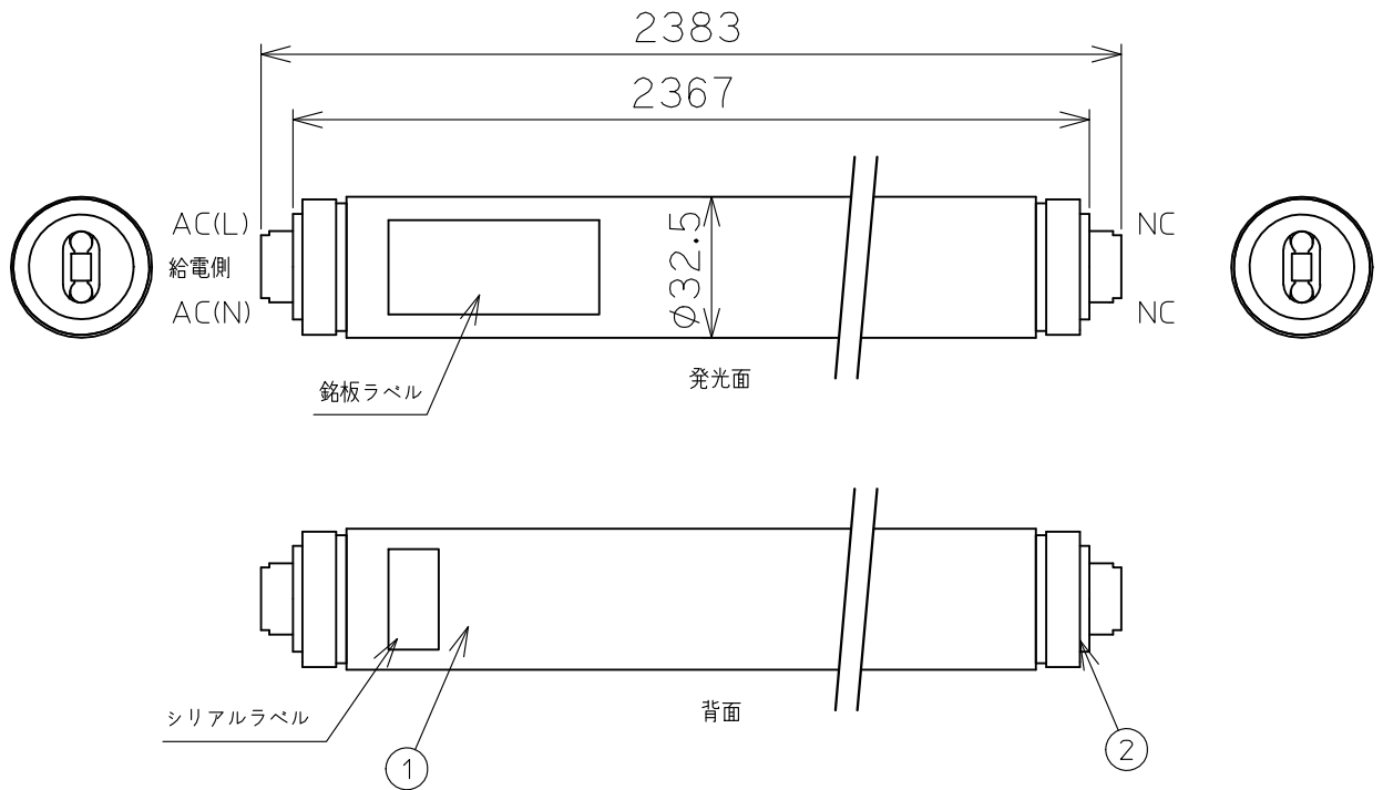
給電端子仕様 (片側給電)
