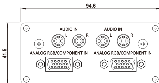
【パネル面】
